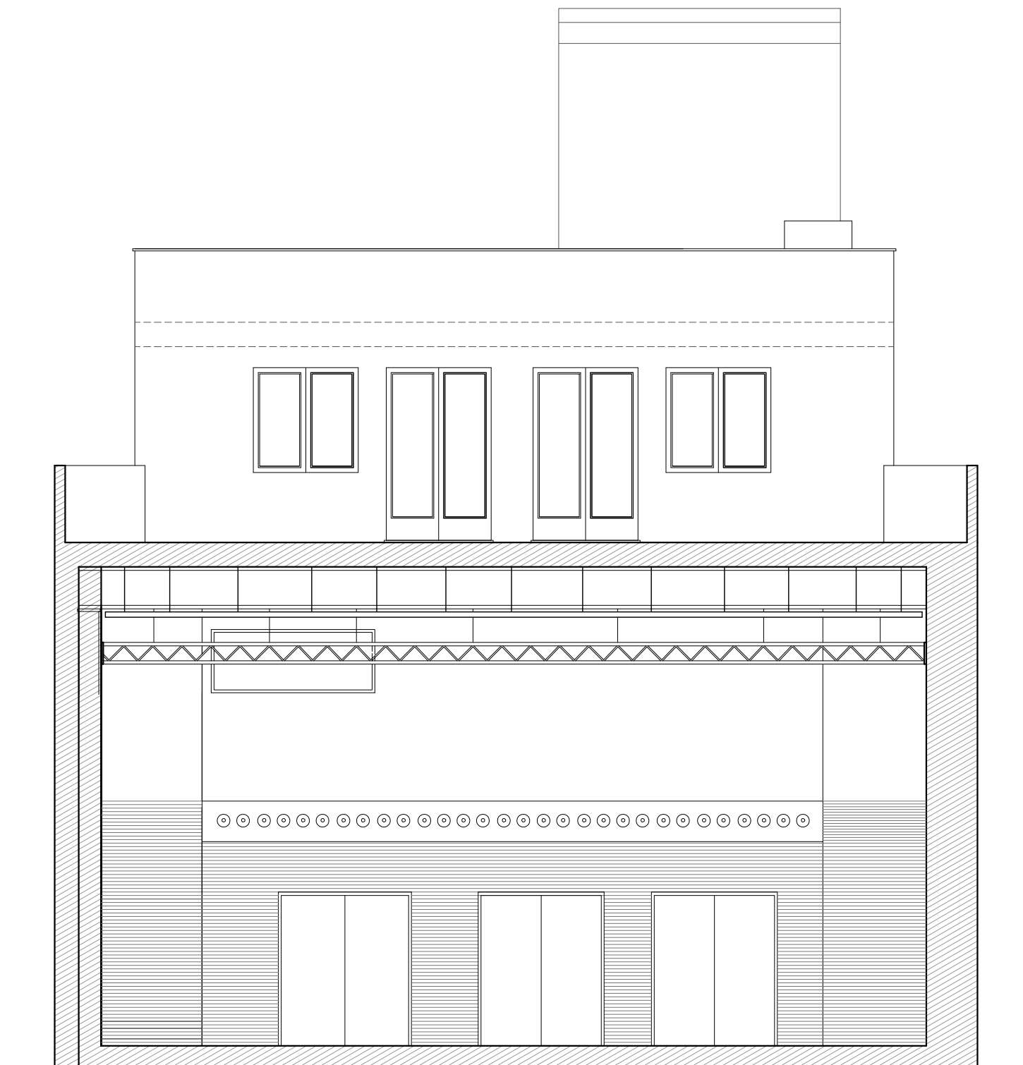
SECCIÓ TRANSVERSAL PER SALA POLIVALENT
